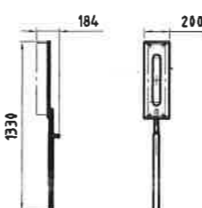
Halter SPAL 2x50,8+2x38 m=11kg
