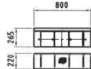
Abdeckung m=19kg
