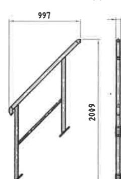
16-Geländer Treppe m=16kg
