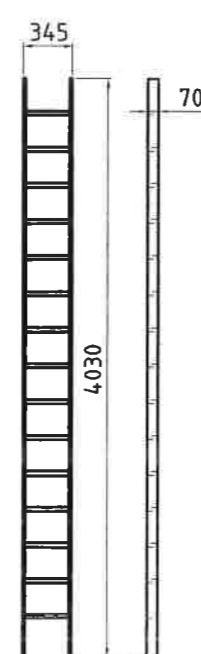
Leiter 2 m=7kg
