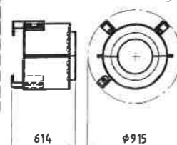
Schutzhaube 2 m=85kg
