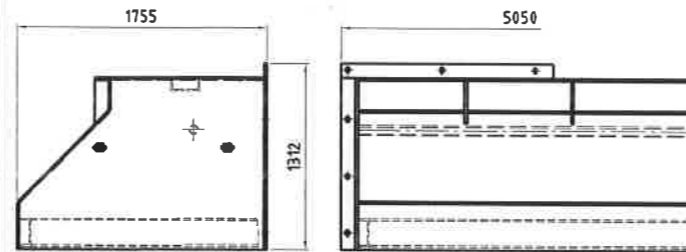
Haube Raupenschiffe m=2733kg
