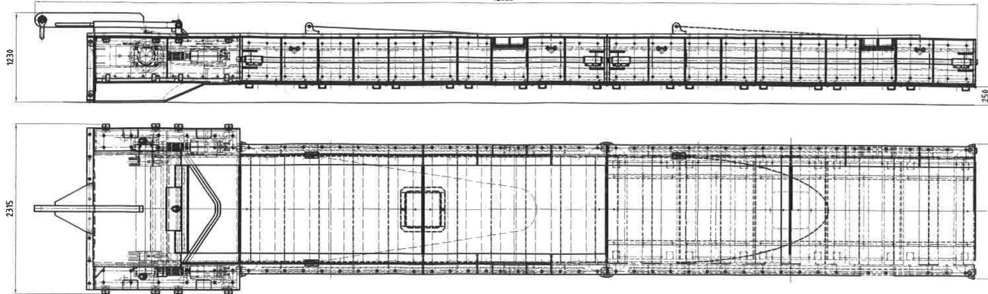
Brechergeh + Walz+Brecherrinne + Antriebsr m=23685kg
