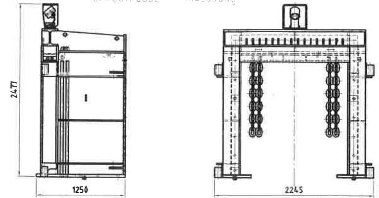
Einlaufhaube m=3850kg
