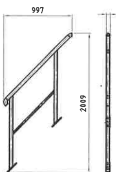
15-Geländer Treppe m=16kg
