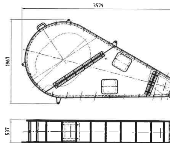
Keilriemenschutzhaube m=970kg
