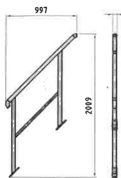
14-Geländer Treppe m=16kg
