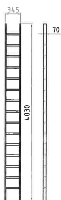
Leiter 1 m=7kg
