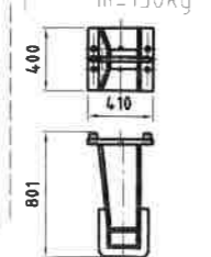
Momentenstütze m=130kg
