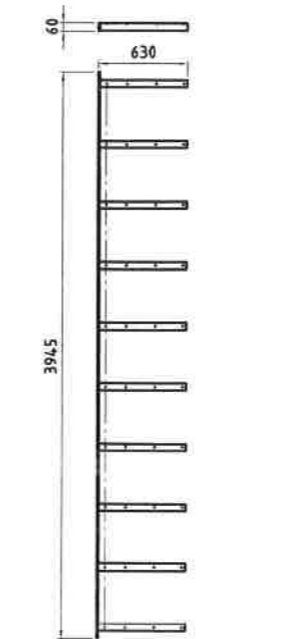
Halter längs m=108kg
