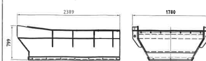
Abwurftrichter m=945kg
