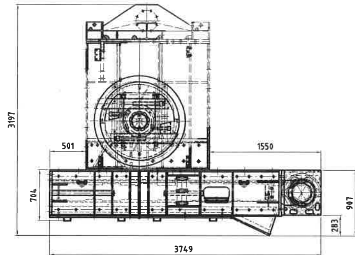
Brechergeh + Walz+Brecherrinne + Antriebsr m=23685kg
