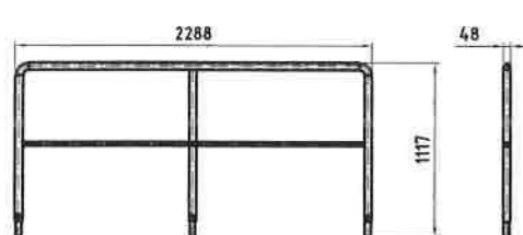
17-Geländer 2x1120 m=23kg
