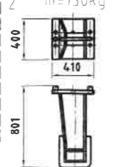
Momentenstütze 2 m=130kg
