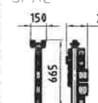
Halter 2 m=34kg SPAL
