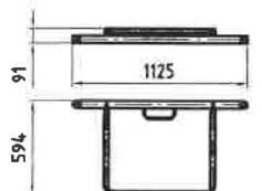
Bügel 1 m=16kg
