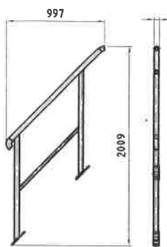
13-Geländer Treppe m=16kg
