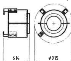
Schutzhaube 1 m=85kg
