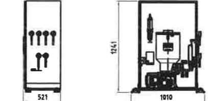
Hydraulikschrank m=130kg
