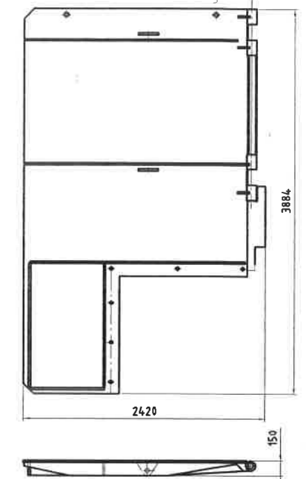
Ausstellbracke rechts m=1407kg
