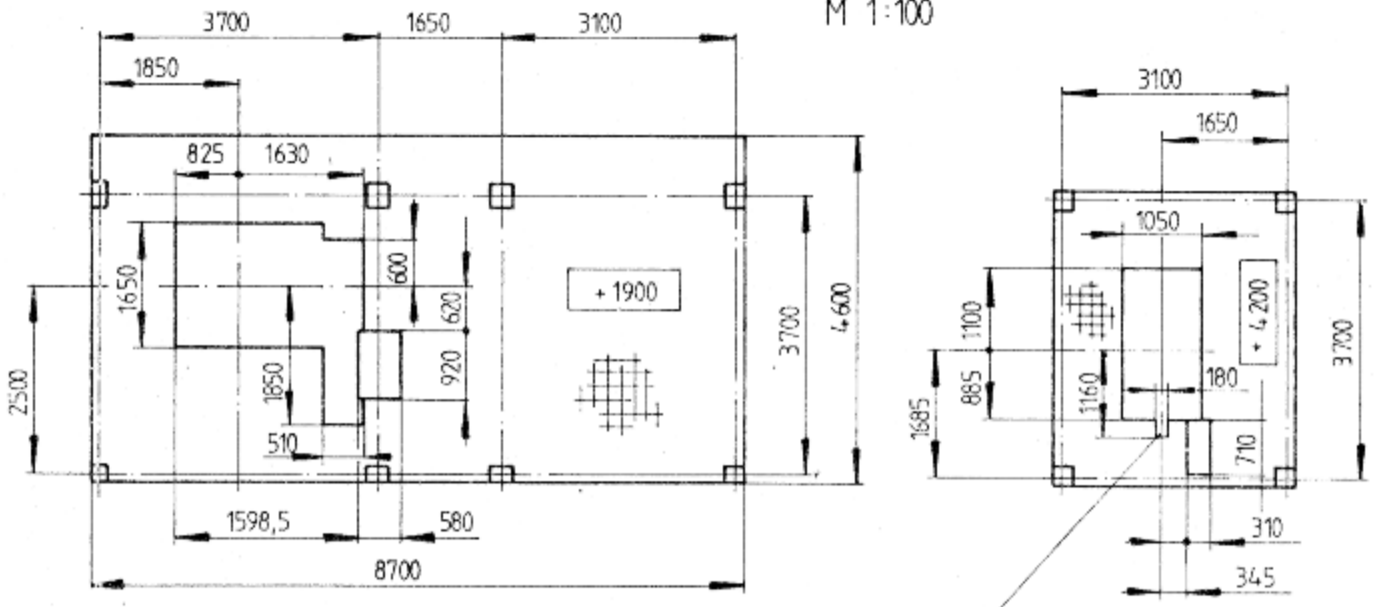
Gitterrostabdeckung M 1:100
