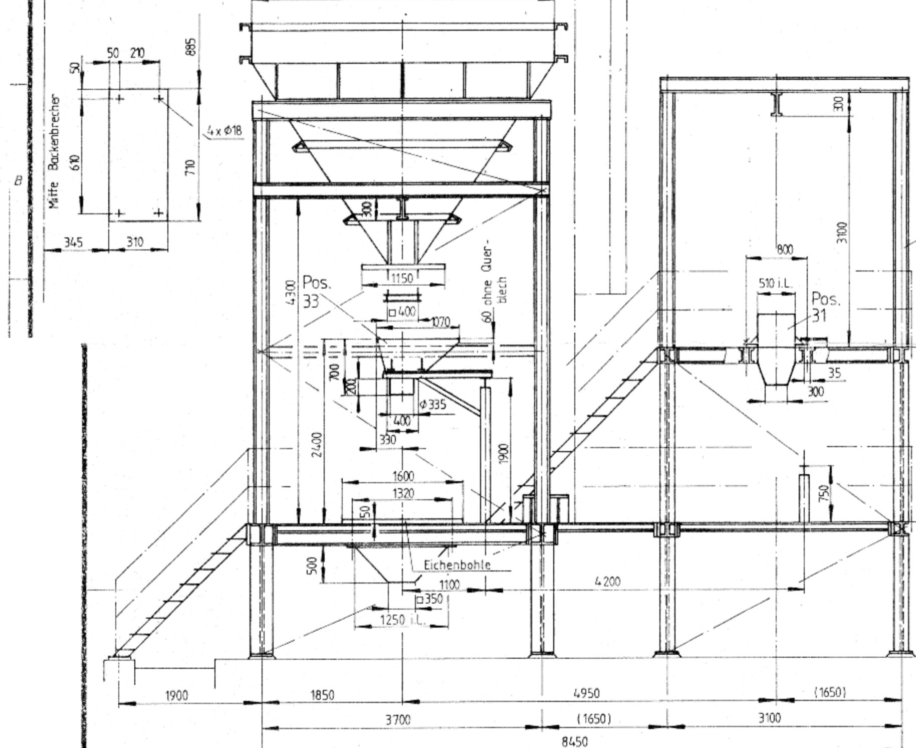
Motorplatte Backenbrecher M 1:20
